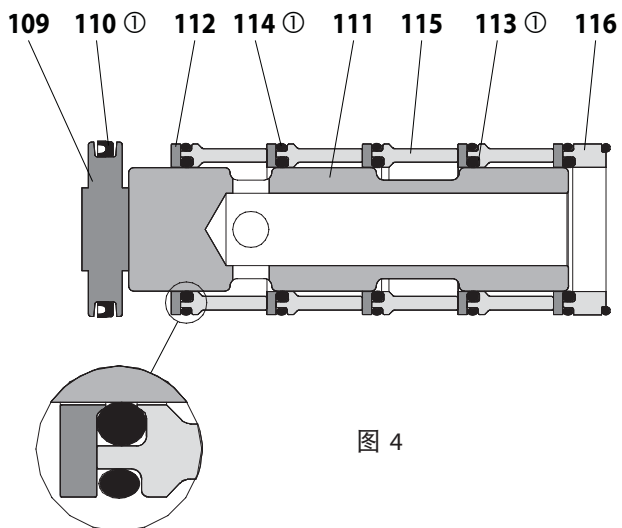
主阀剖视图
